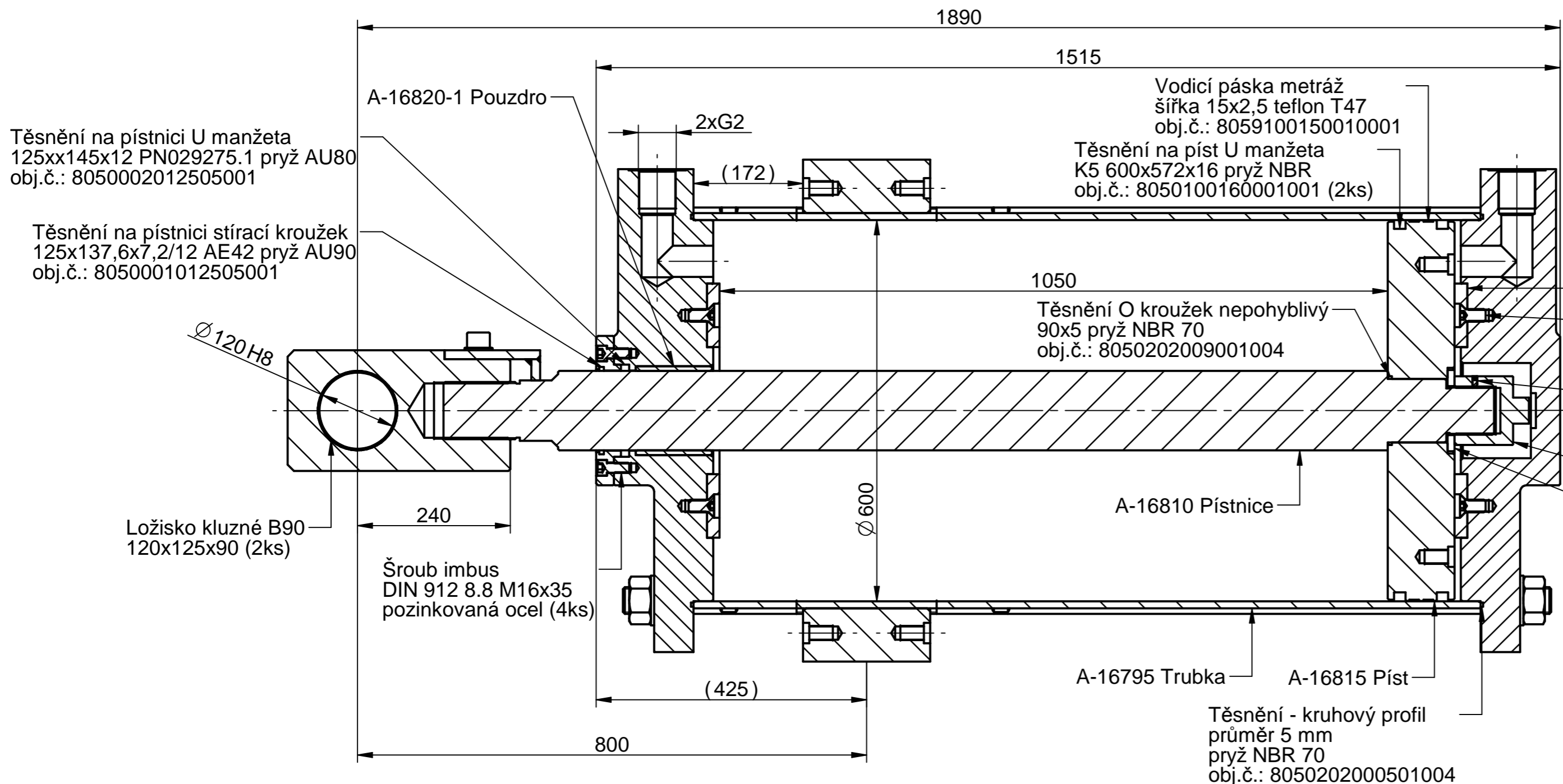
ŘEZ A-A
